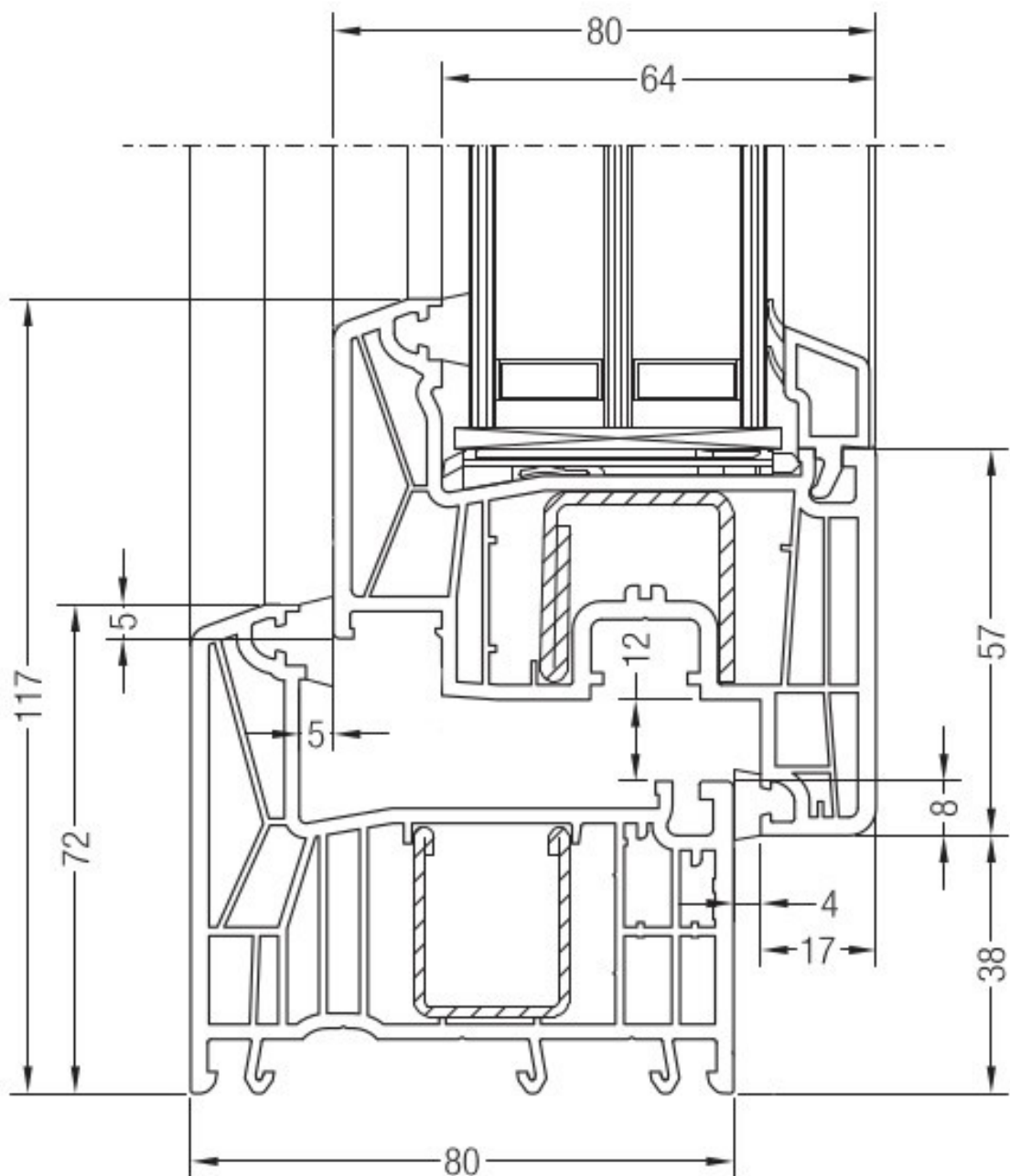
řez rámu a křídla
