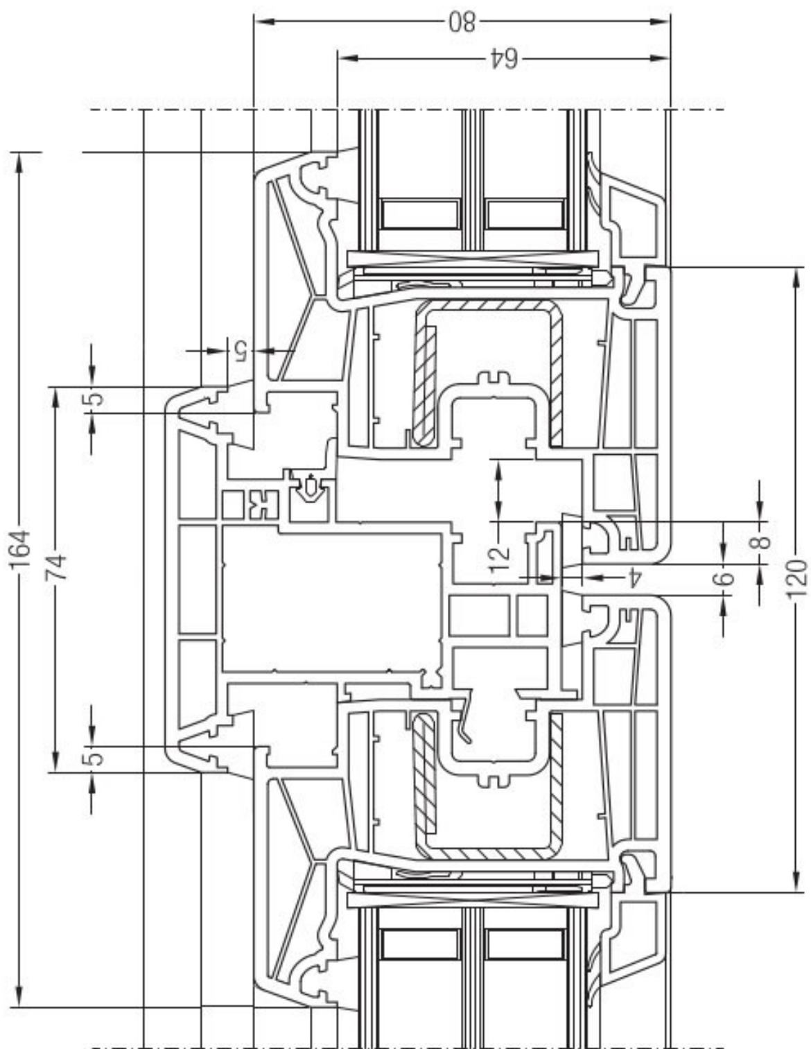
řez křidel a štolpu
