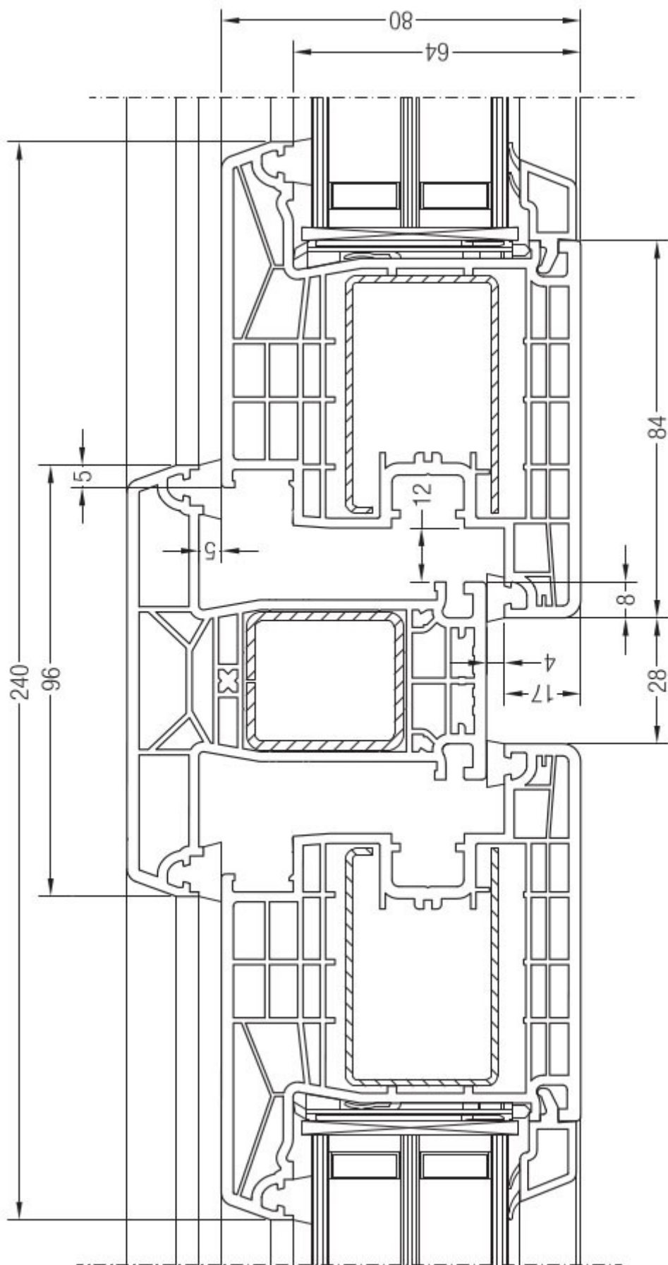
řez křidel a sloupku
