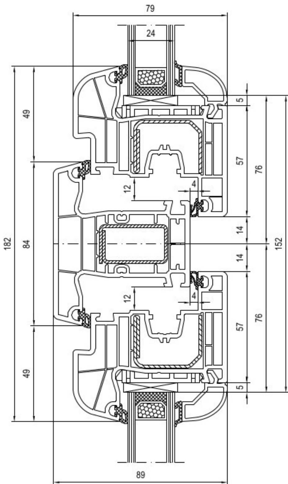
řez křídel a sloupku
