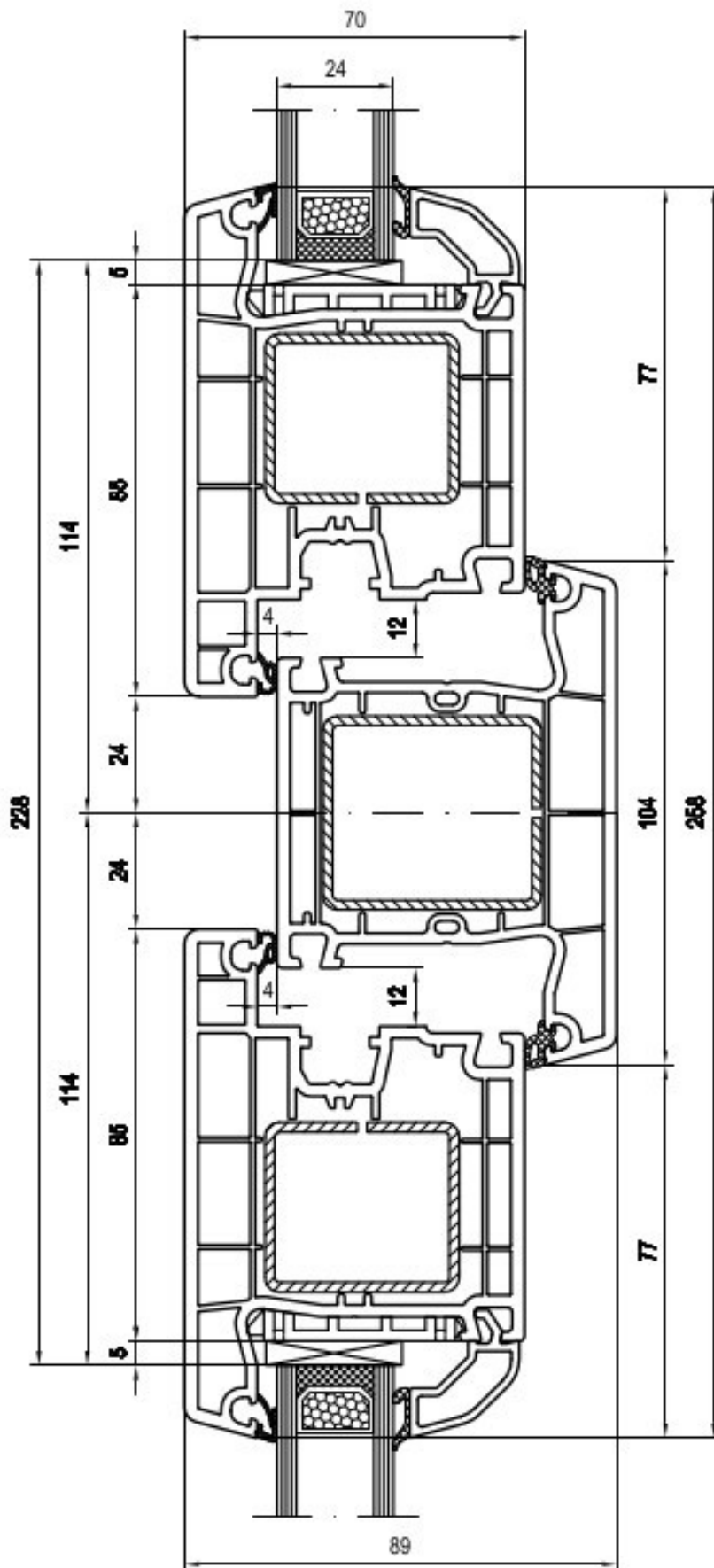
řez křídla a sloupku
