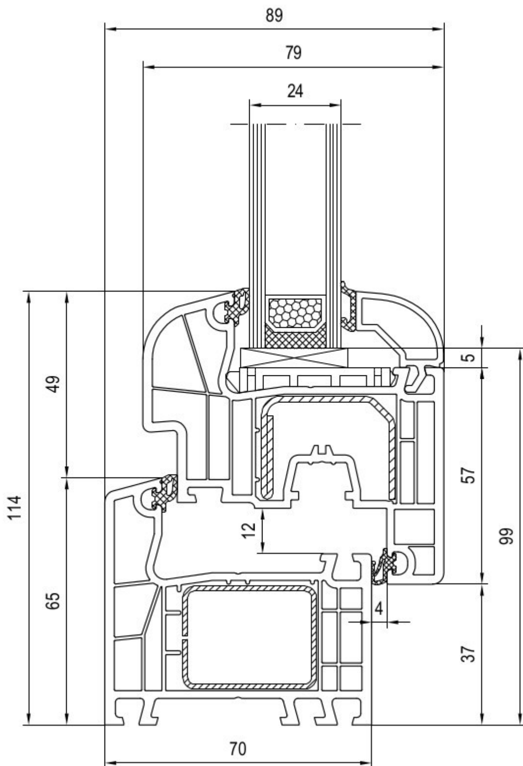
řez rámu a křídla
