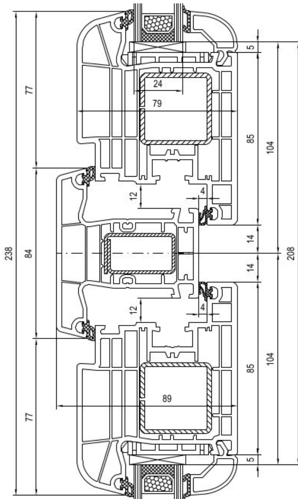
řez křídel a sloupku
