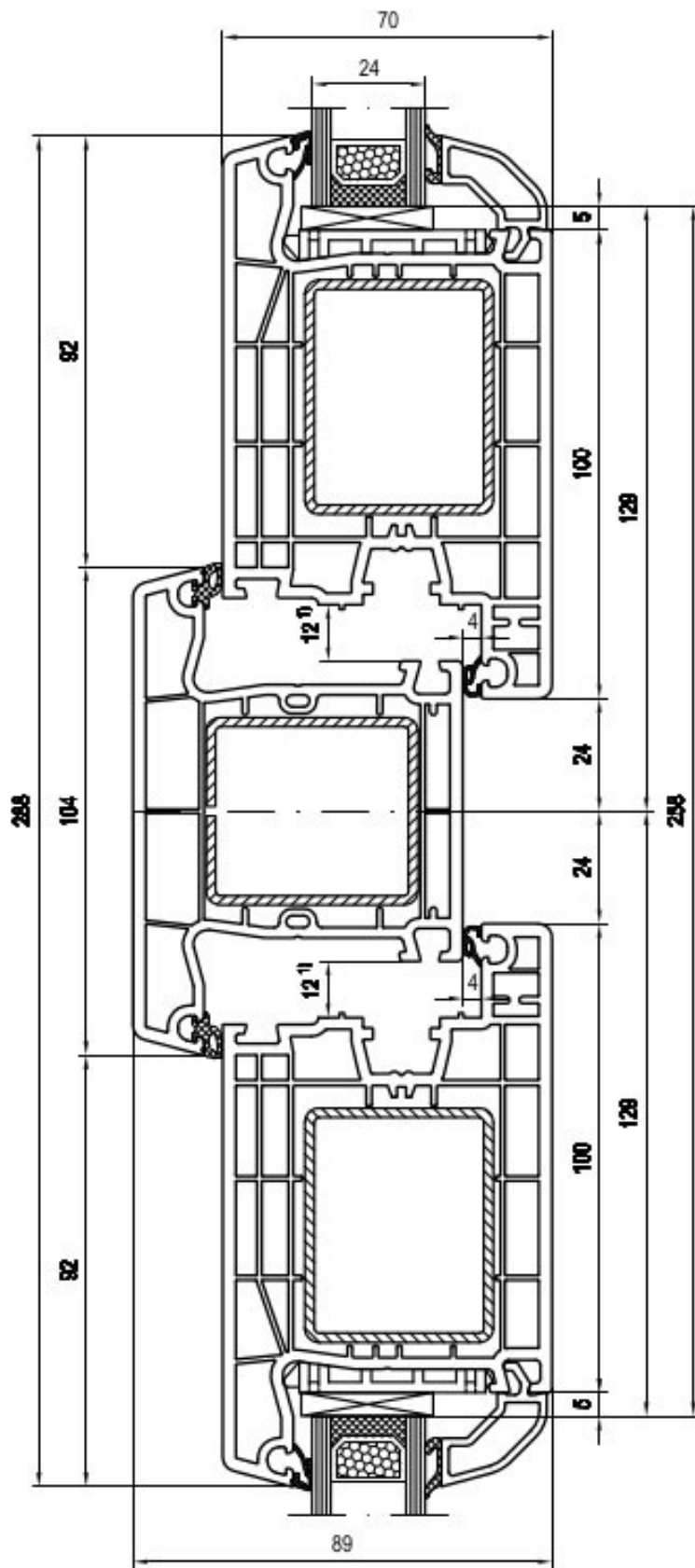
řez křidel a sloupku
