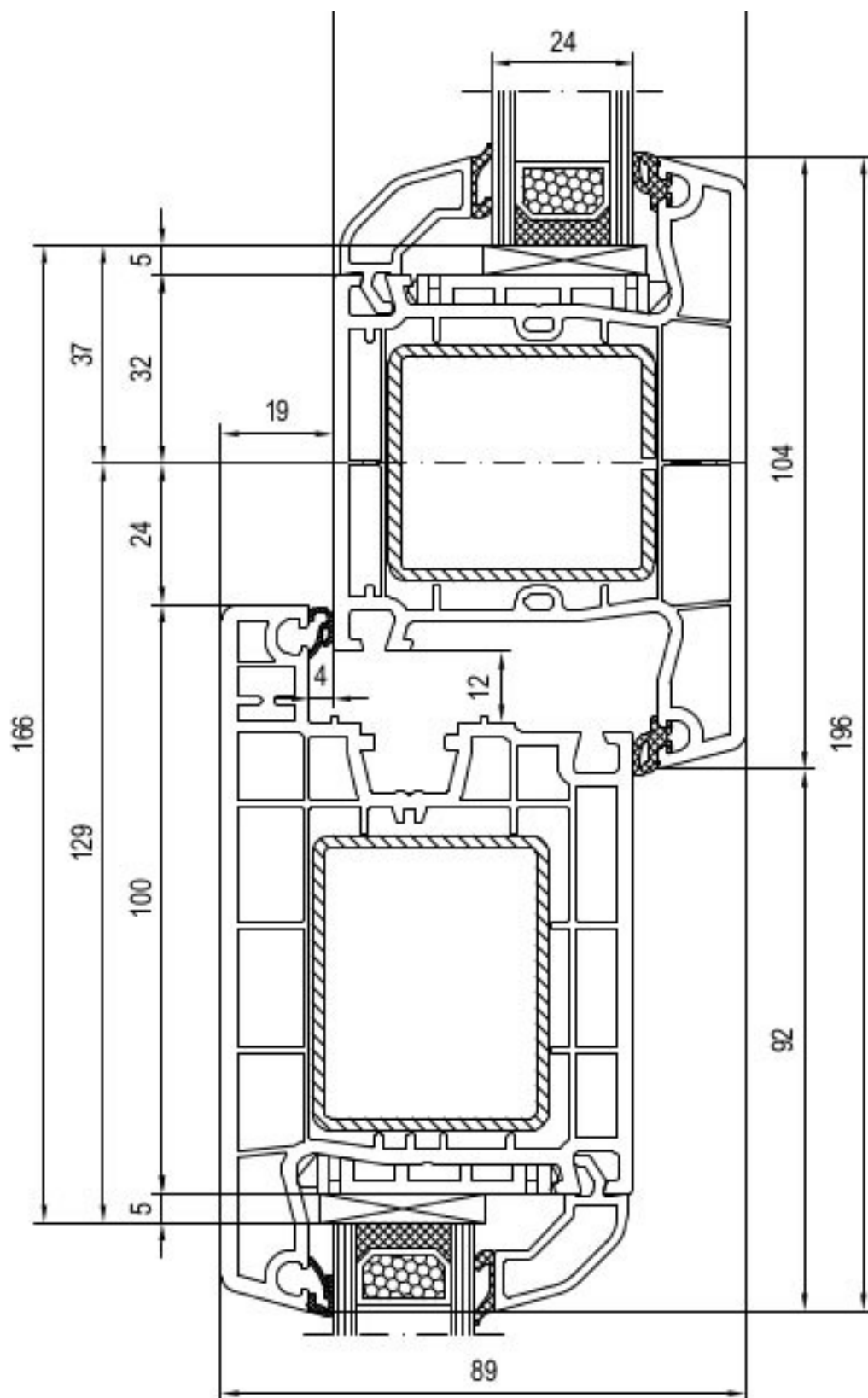
řez křídla a sloupku
